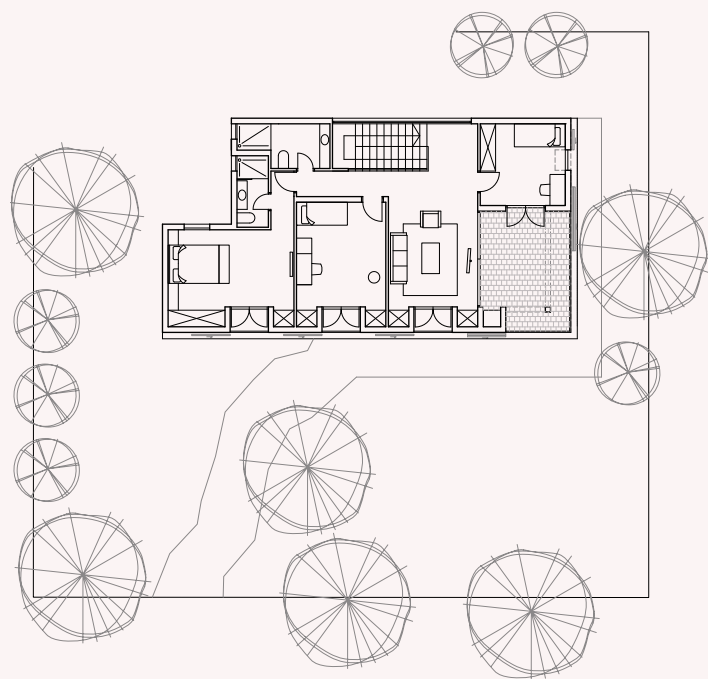
תכנית העמדה - קומה ראשונה
